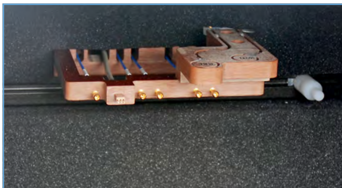
Prüflingskontaktierung
