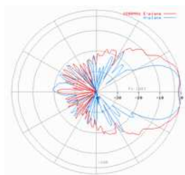
2200 MHz
