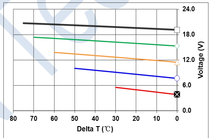
Performance Curves Th=50 °C (性能曲线 Th=50°C)
