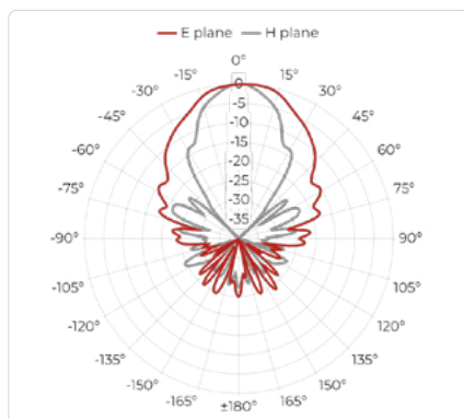
Port B, 16 GHz
