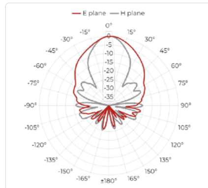
Port B, 18 GHz
