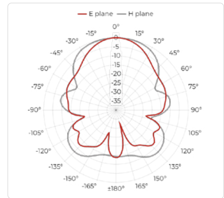
Port B, 8 GHz
