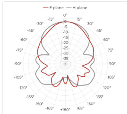
Port B, 10 GHz
